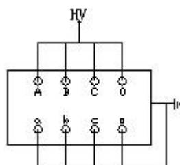
图 6-10 变压器反接法
