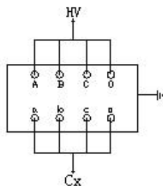
图 6-9 变压器正接法
