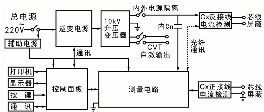
图 2—1 测量原理图
