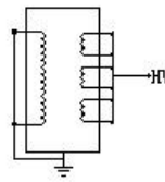
图 6-3 PT 接法
