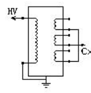
图 6-4 PT 末屏法
